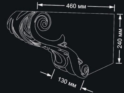
Цоколь МДФ №2
